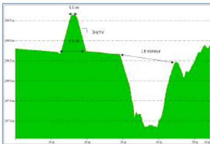
Figure 4 : Emprise de la digue sur le linéaire amont (secteur aval : PM : 75)
