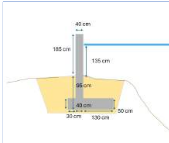
Figure 5 : Murs de protection contre les inondations
