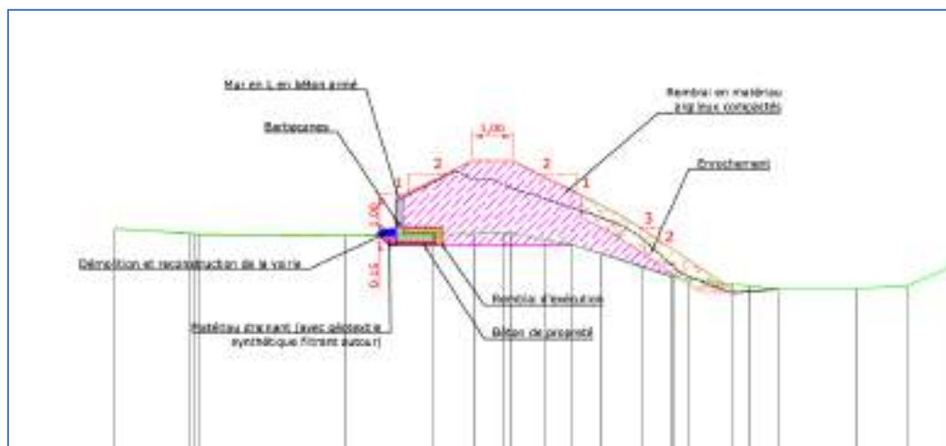
Figure 6 : coupe ouvrage état AVP
