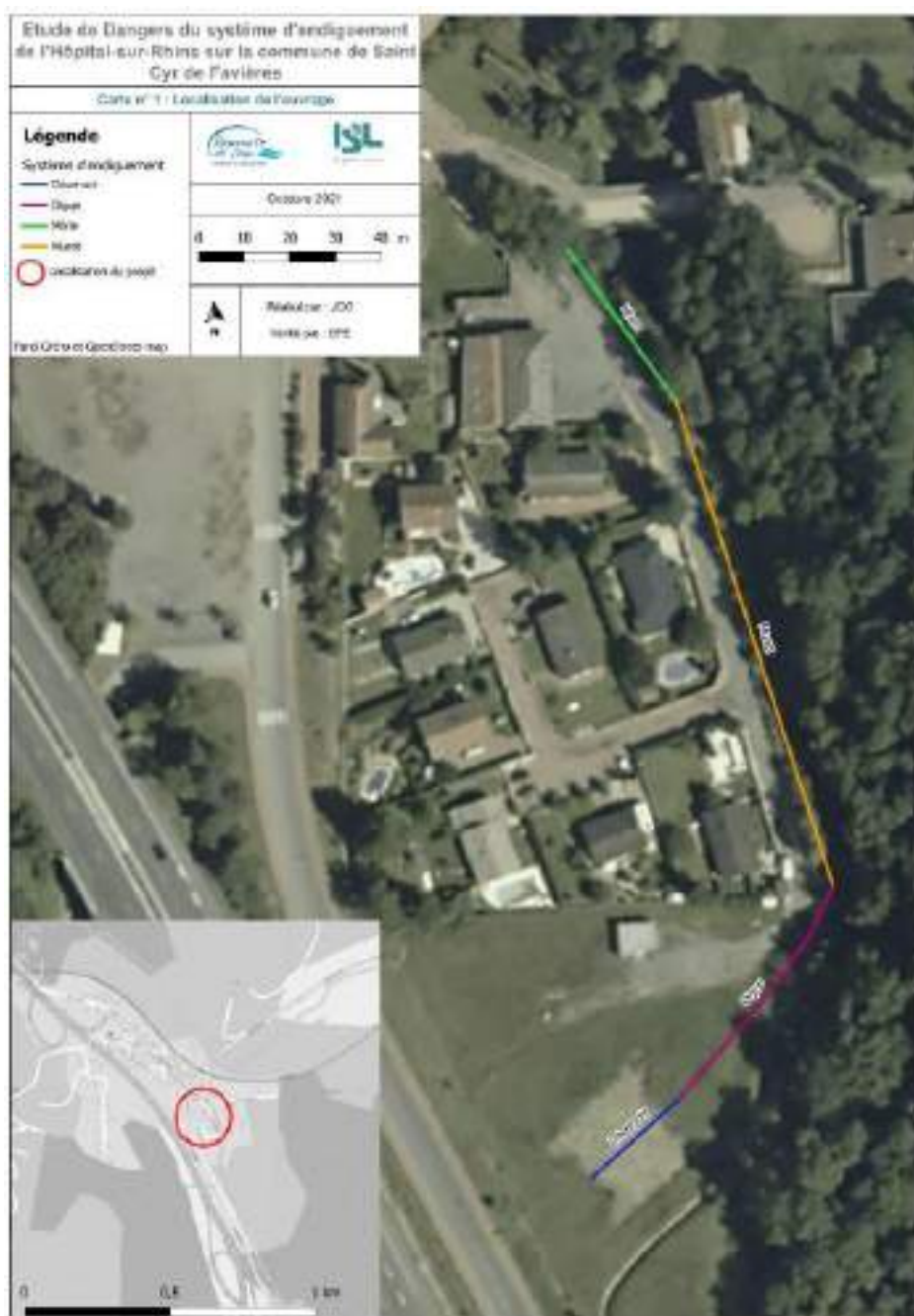
Figure 1 : tronçons homogènes et ouvrages du système d'endiguement actuel
