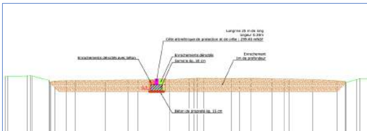
Figure 2 : Schéma de principe du déversoir
